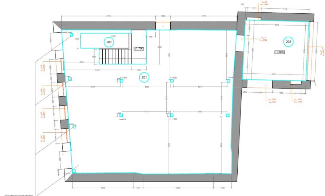
Экспликация помещений 1 этаж
